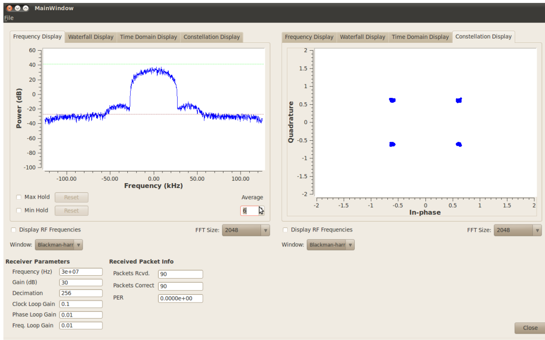
Figura 4-11: Constelación observada al transmitir un archivo a 30kbit/s.
