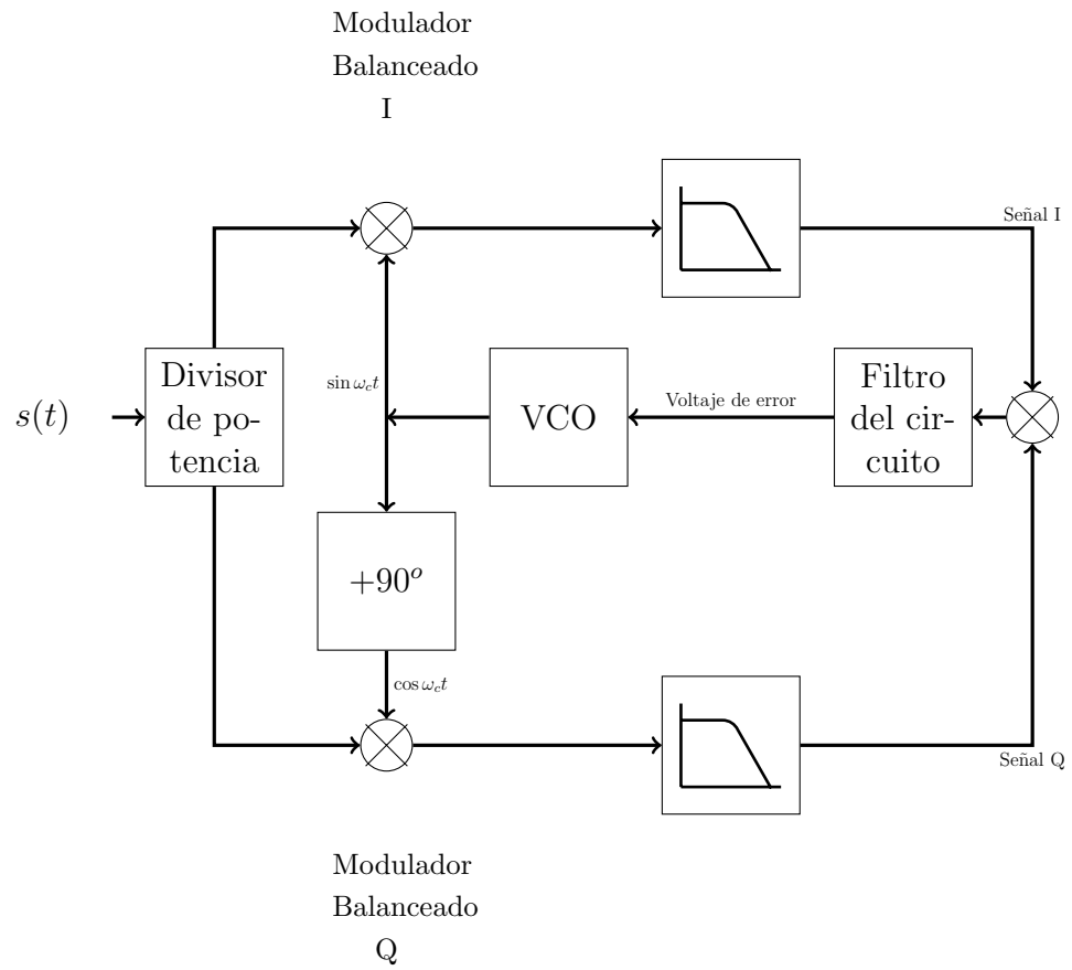
Figura 2–12: Diagrama a bloques de un sincronizador de Lazo de Costas. (Pérez, 2004)
