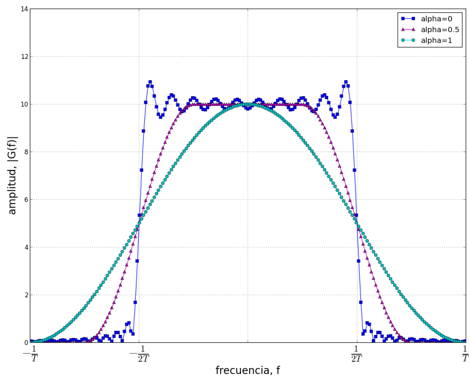
Figura 3–12: Representación en el dominio de la frecuencia de filtros coseno elevado
