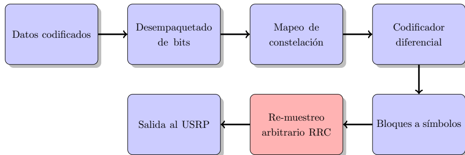
Figura 3–16: Estructura del modulador DQPSK con filtros polifásicos
