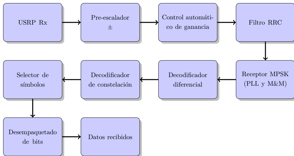
Figura 3-18: Estructura del demodulador DQPSK
