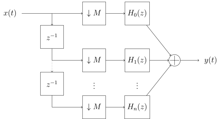
Figura 3–15: Descomposición del filtro decimador en su representación polifásica (Farhang, 2010).
