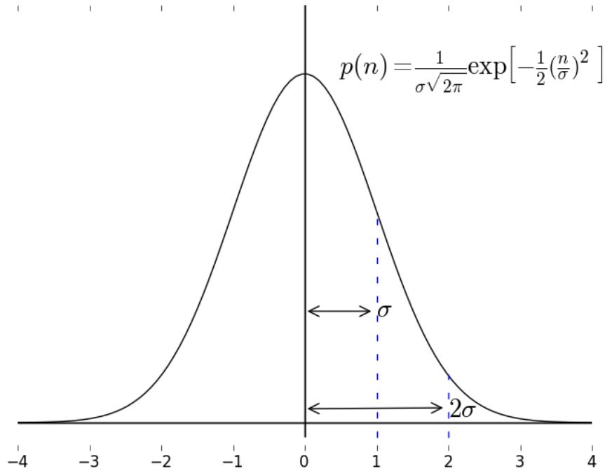
Figura 2–3: Función de densidad de probabilidad de la distribución Gaussiana ( Sklar, 2001 )
