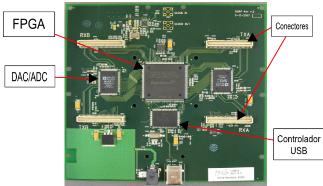
Figura 3-1: Placa principal del dispositivo USRP.
