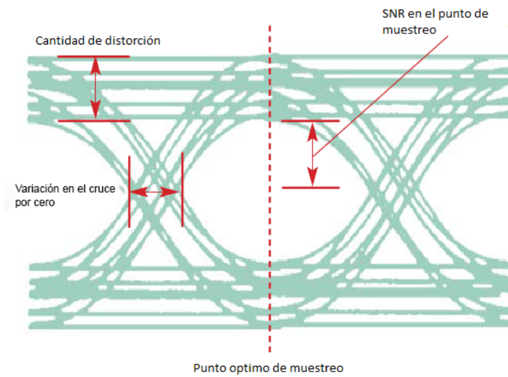
Figura 2–9: Parámetros de medición de un diagrama de ojo.
