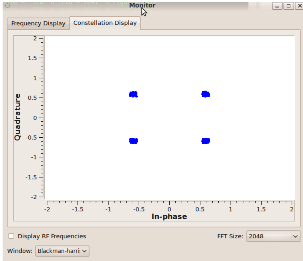
Figura 4-9: Constelación obtenida con parámetros óptimos de una transmisión a 100kbts/s
