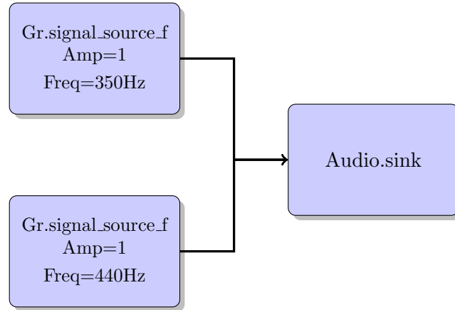
Figura 3–6: Grafo que envía dos senoidales a la tarjeta de audio de una PC.
