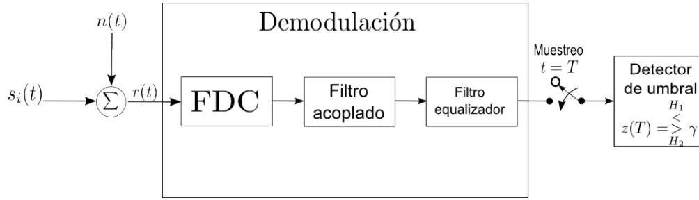
Figura 2-4: Diagrama simple de un demodulador digital.
