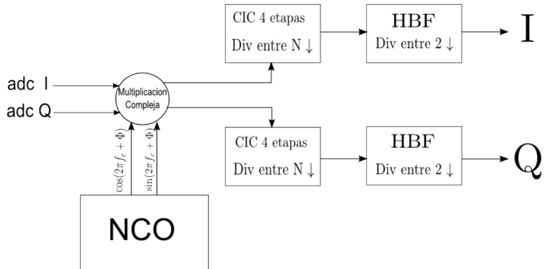
Figura 3–2: Estructura de un DDC implementado en el USRP
