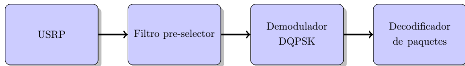
Figura 3-17: Diagrama a bloques del receptor DQPSK
