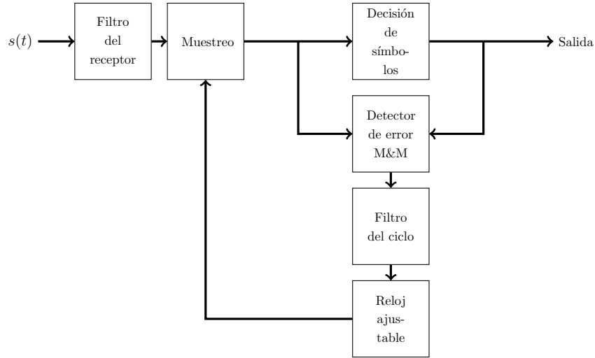
Figura 2–13: Diagrama a bloques del sincronizador M&M. (Meyr, 1998)
