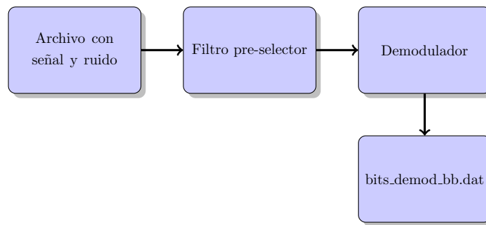
Figura 4-3: Grafo que realiza la demodulación de la señal simulada
