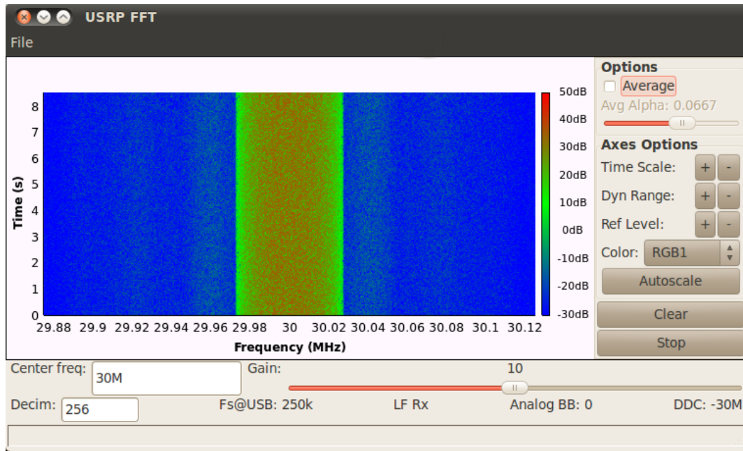
Figura 4–8: Aplicación en Python que muestra el espectrograma de lo que el USRP está capturando.
