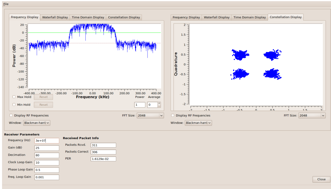
Figura 4-8: Resultados de la transmisión con parámetros por defecto del programa a 100kbts/s.
