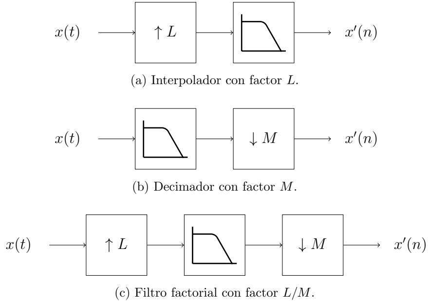
Figura 3–14: Estructuras básicas de filtros multi tasa (Farhang, 2010).
