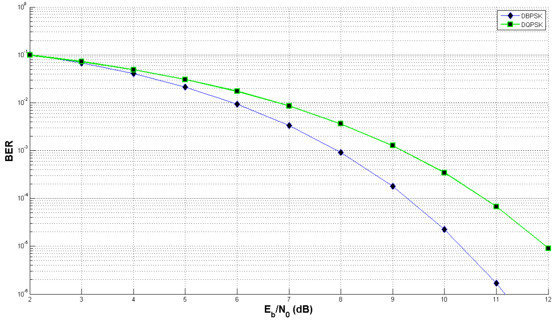
Figura 4-7: Resultados teóricos de la herramienta BERTool de Matlab.
