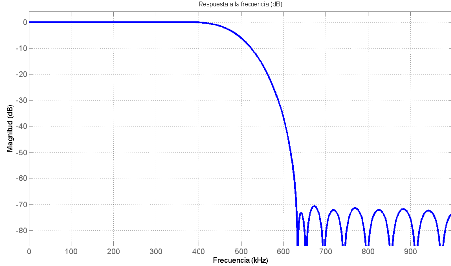
Figura 3-4: Respuesta a la frecuencia del filtro de media banda
