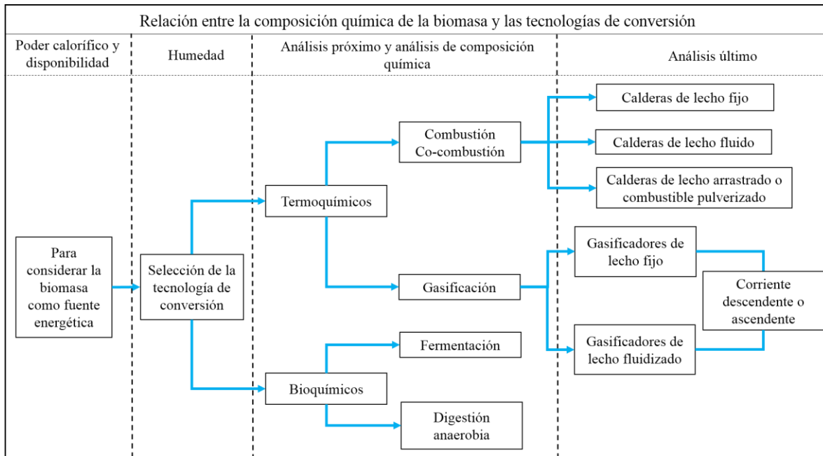
Figura 19. Relación entre análisis de caracterización y tecnologías de conversión.
