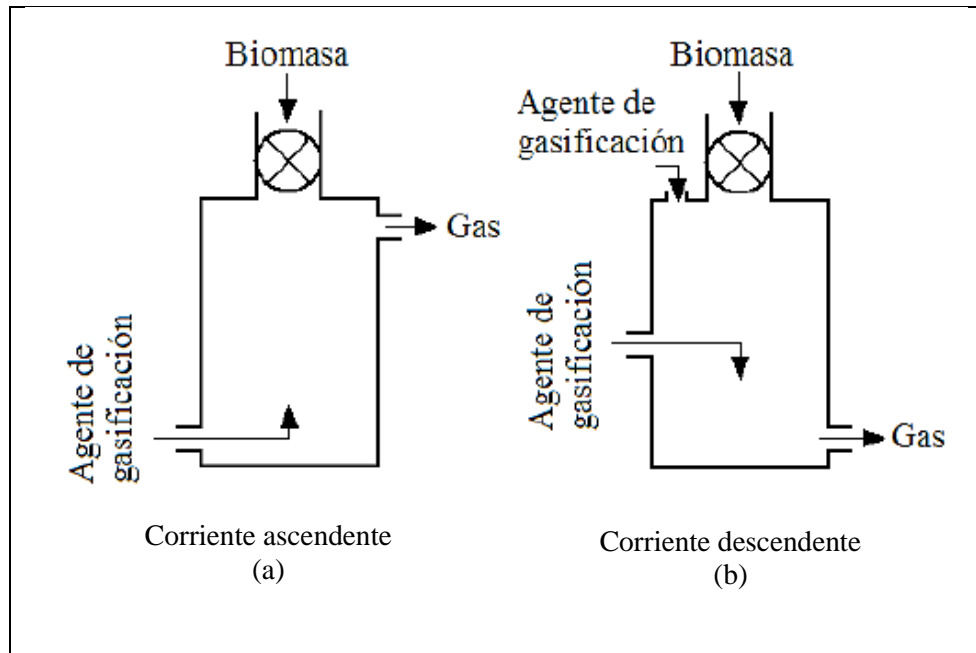
Figura 17. Gasificadores de flujo a) ascendente, (b) descendente [5].
