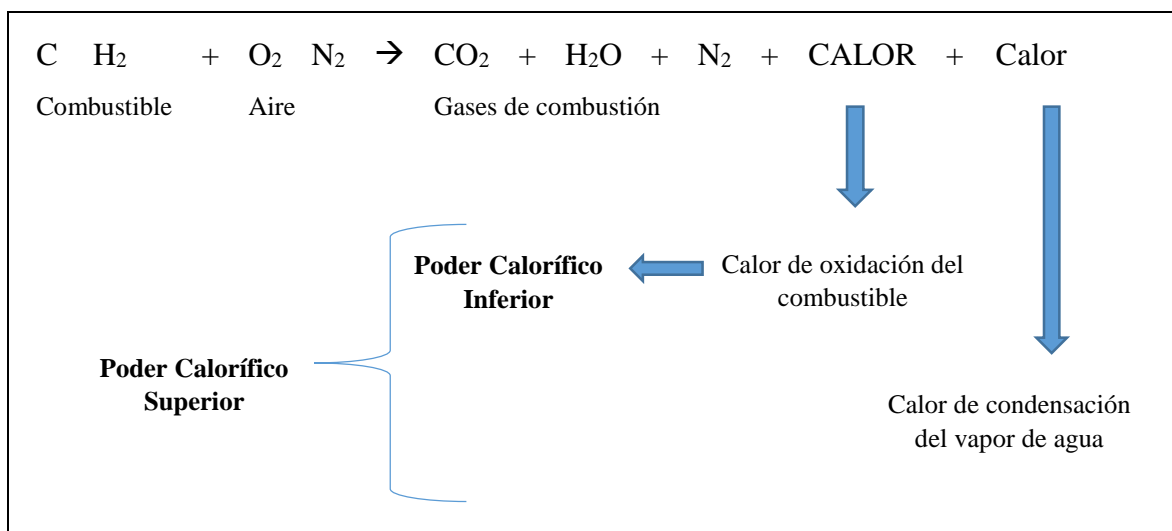
Figura 8. Diferencia entre PCS y PCI.
