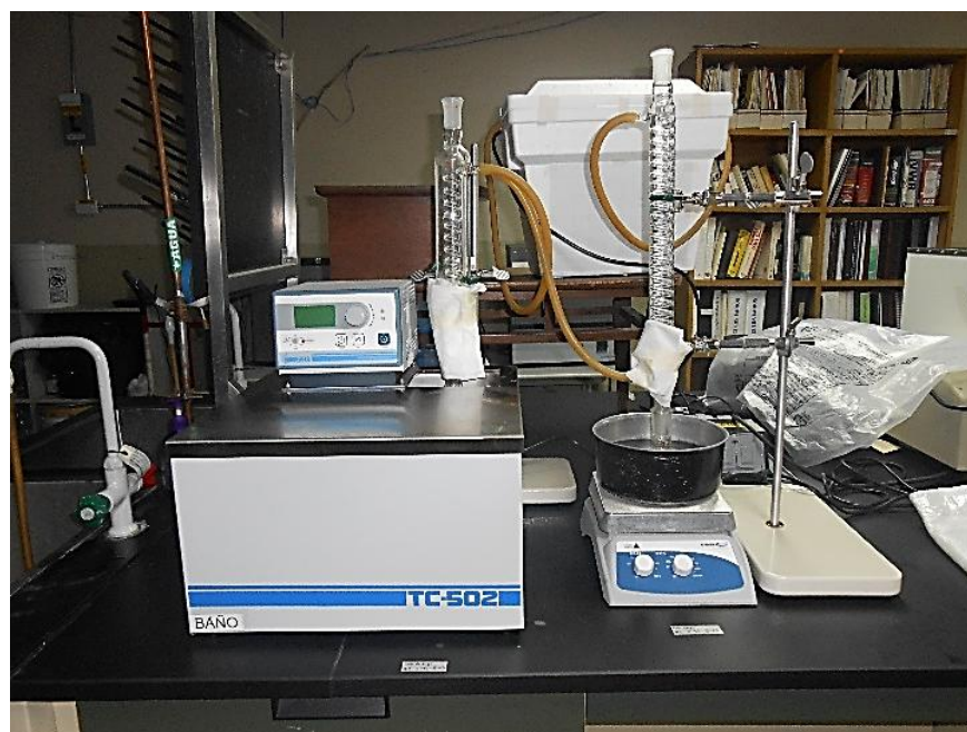
Figura 28. Extracción en agua caliente.
