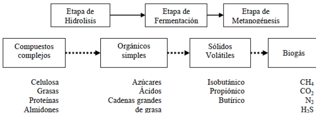
Figura 18. Proceso de digestión anaeróbica [10].
