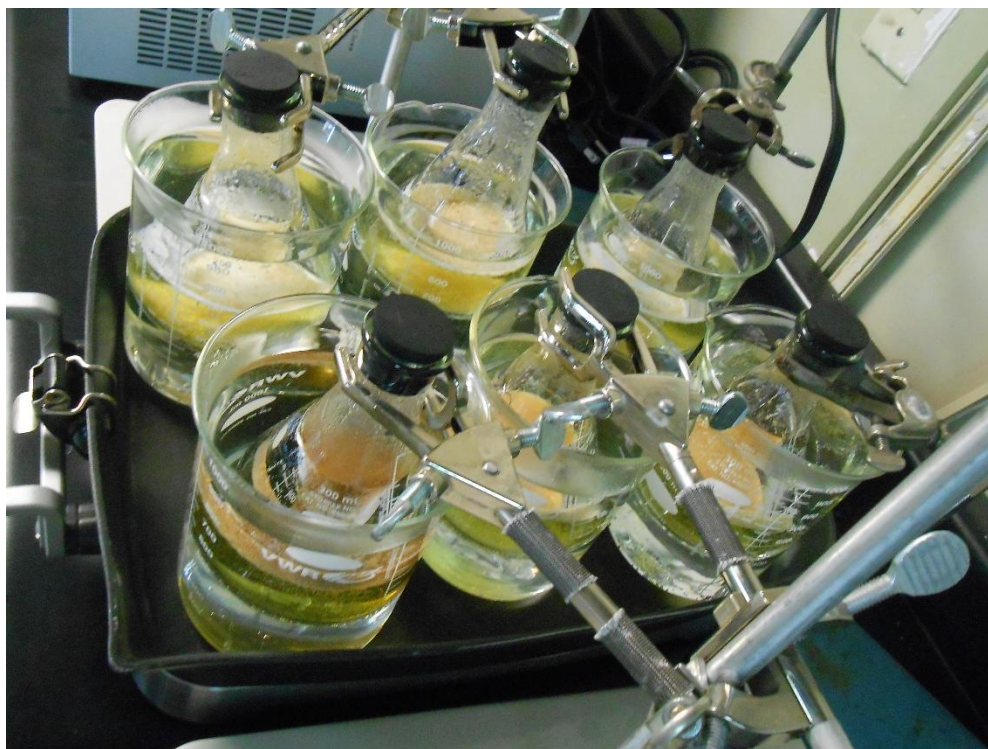
Figura 31. Montaje para la determinación del porcentaje de Holocelulosa.
