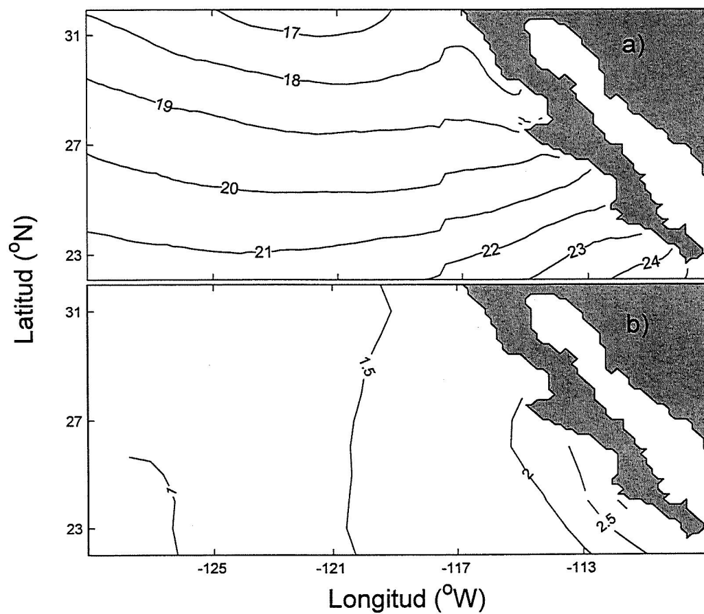
Figura 5. a) Distribución horizontal del promedio total de la TSM (en ^{\circ}\text{C} ). b) Desviación estándar del promedio total. Ambos, generados a partir de 17 años de información.
