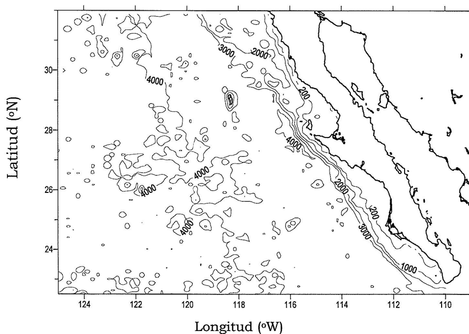
Figura 4. Batimetría de la zona de estudio. Las profundidades se muestran en metros.
