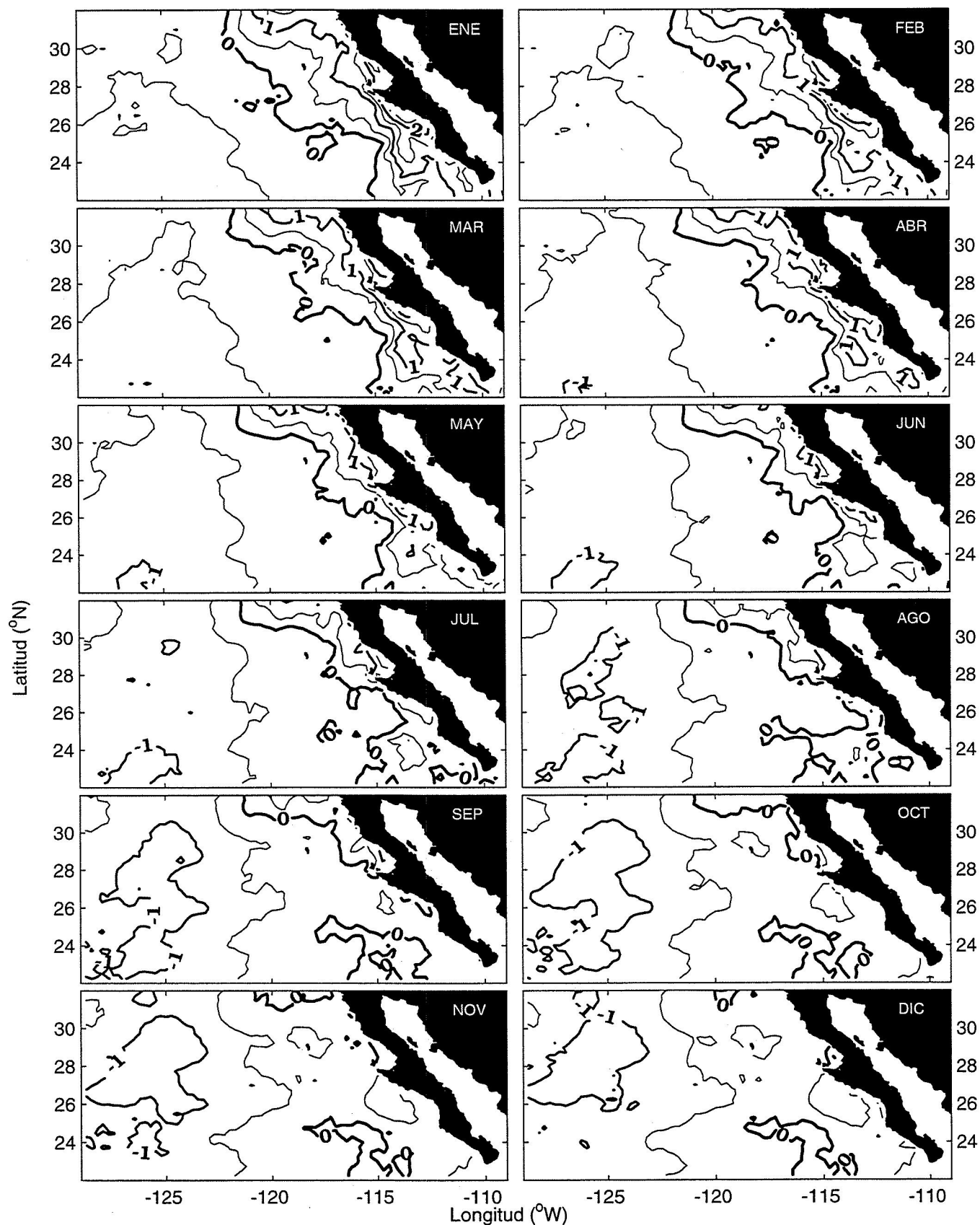
Figura 14.2- Anomalías térmicas interanuales para 1984
