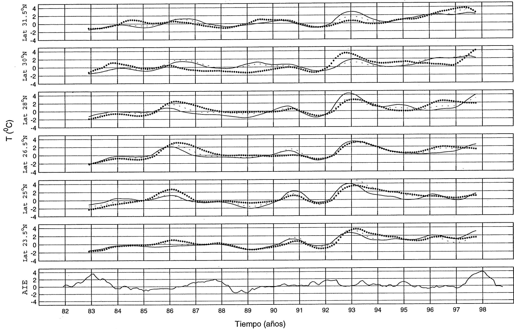
Figura 13. Series de tiempo de las anomalías termales interanuales, mostrando la comparación entre las zonas oceanográfica(o), transicional(-- y costera(-) y la anomalía interanual registrada en el ecuador por la NOAA (AIE).
