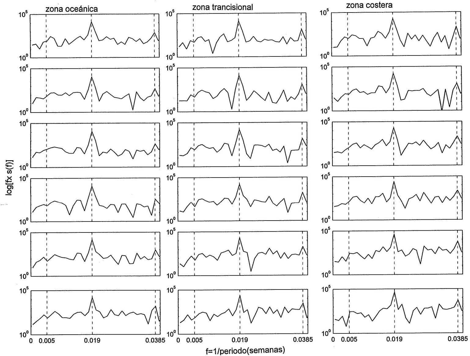
Figura 9. Espectros de potencia para las series originales. El eje de las ordenadas representa el logaritmo base 10 de la multiplicación de la frecuencia por las serie de fourier. El valor de frecuencia f=0.005 representa 3.84 años, f=0.019 representa 1 año, f=0.0385 representa 6 meses
