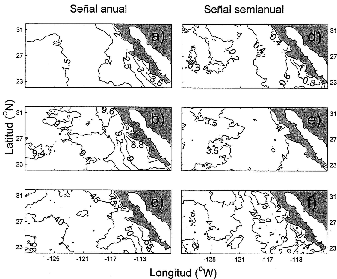
Figura 12. Análisis armónico. Distribución de la amplitud (a y d), fase (b y e) y porcentaje de varianza explicada. El valor de fase representa el mes en que la amplitud es mayor. Ejemplo: septiembre=9, abril=4, etc. Nota: En el análisis de la señal anual, se utilizaron las series promediadas semanalmente y en la semianual, la series promediadas mensualmente.
