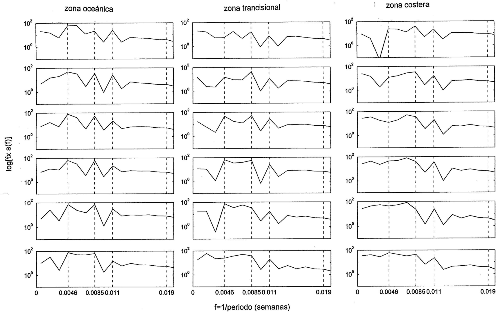
Figura 10. Espectros de potencia para las series interanuales. El valor de frecuencia f=.0046 representa 4.18 años, f=.0085 representa 2.25 años f=.011 representa 1.74 años y f=.019 representa la señal anual
