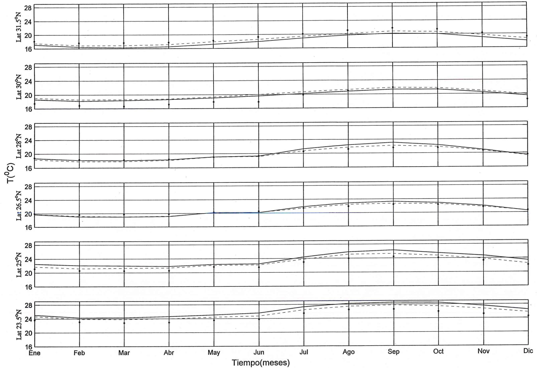
Figura 8. Oscilación promedio de la TSM, mostrando la comparación entre las zonas oceanográfica(o), transicional(--), y costera(-).
