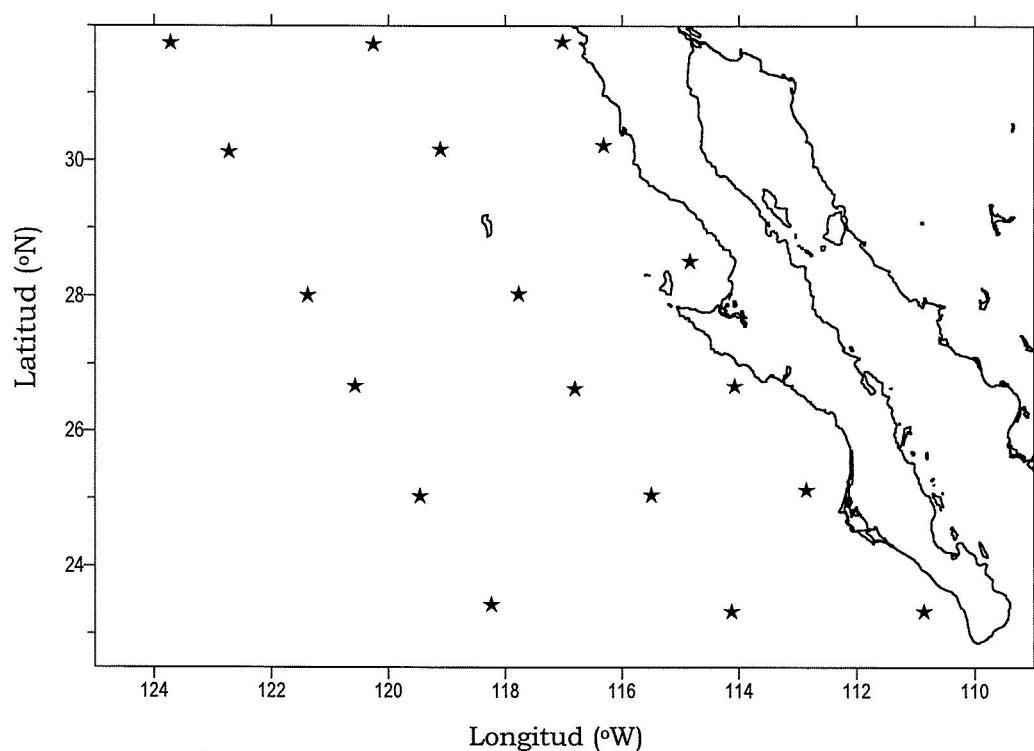
Figura 3. Área de estudio. Los símbolos (★) indican las posiciones de las celdas, que se utilizaron para observar los resultados del análisis de densidad espectral y la comparación entre algunas series de tiempo (tanto semanales como de anomalía interanual).
