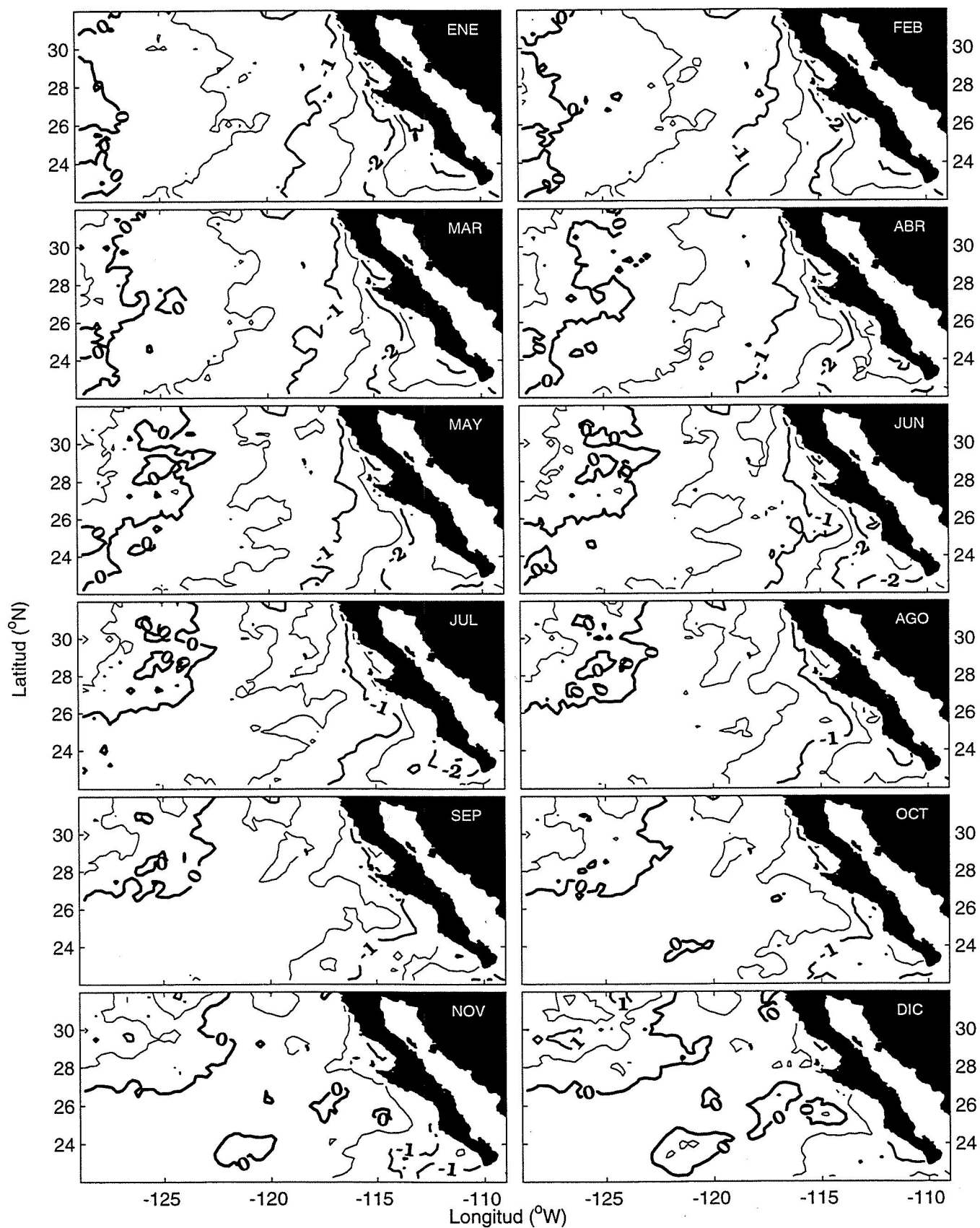
Figura 14.6- Anomalías termales interanuales para 1989
