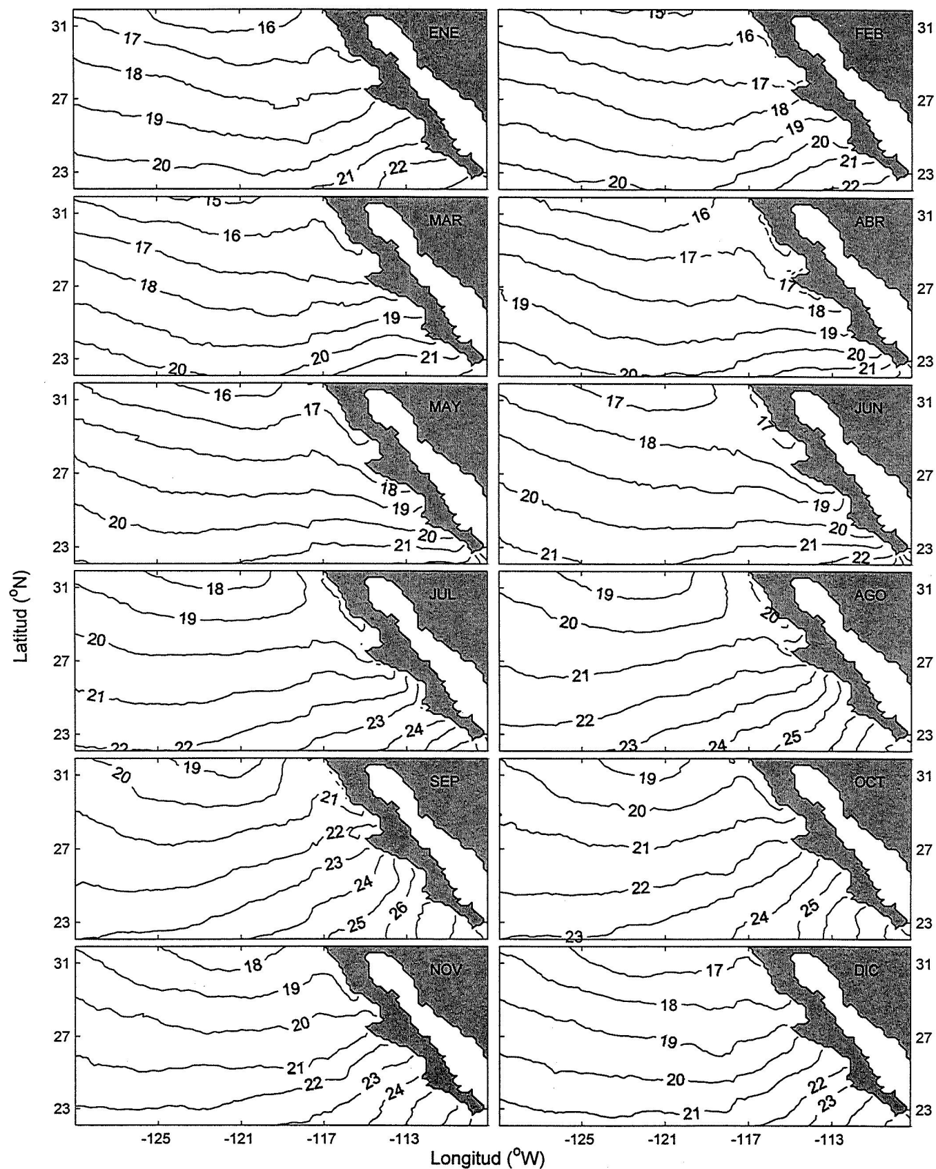
Figura 6. Distribución horizontal del Promedio Climatológico Mensual, para la TSM.
