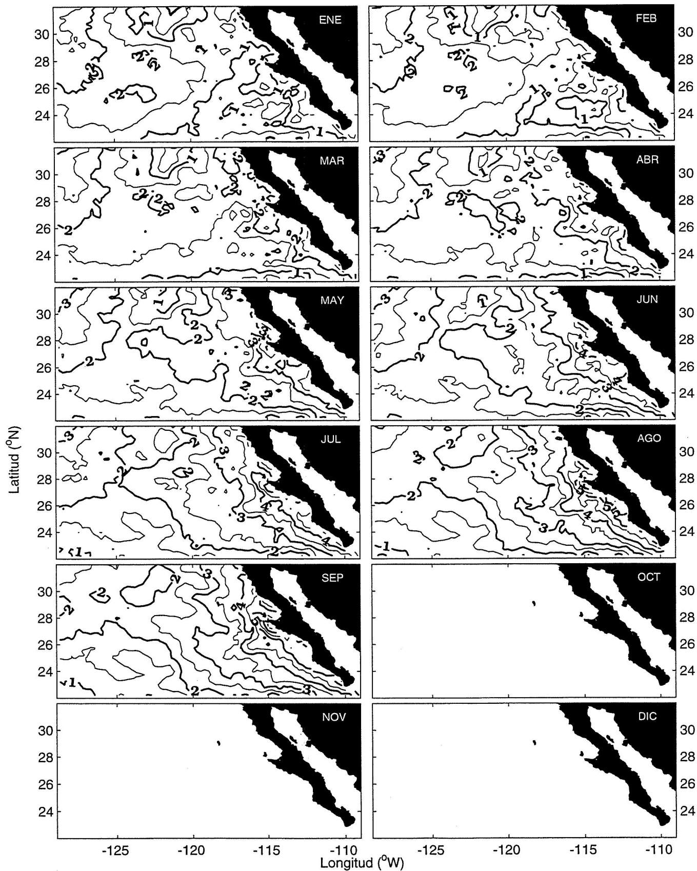
Figura 14.10- Anomalías termales interanuales para 1997
