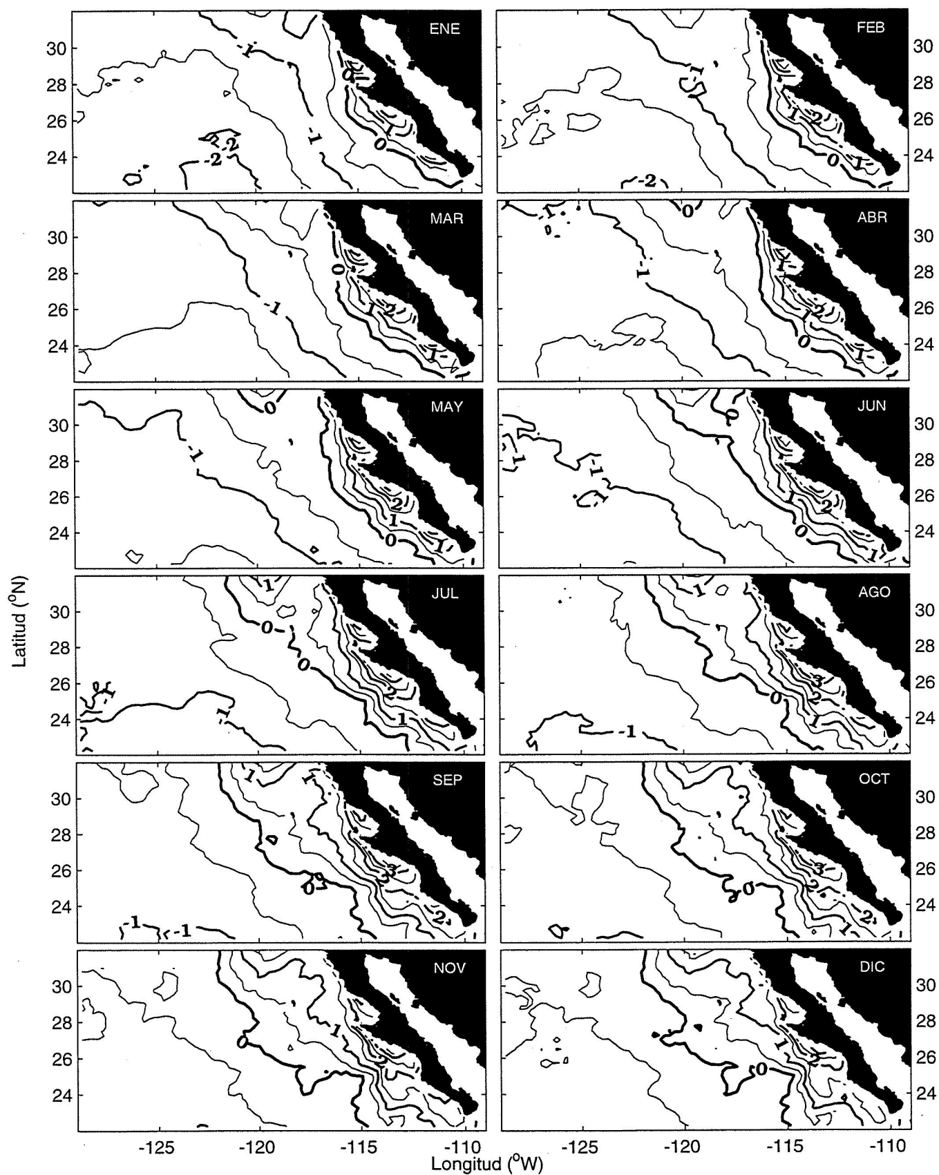
Figura 14.1- Anomalías térmicas interanuales para 1983
