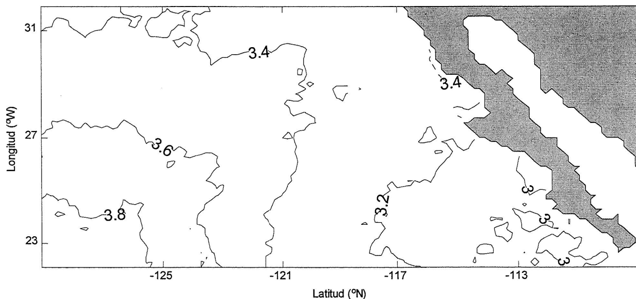
Figura 11. Distribución horizontal de la autocorrelación RTT (t). El valor representa el número de meses que tarda la TSM en cambiar de temperatura.
