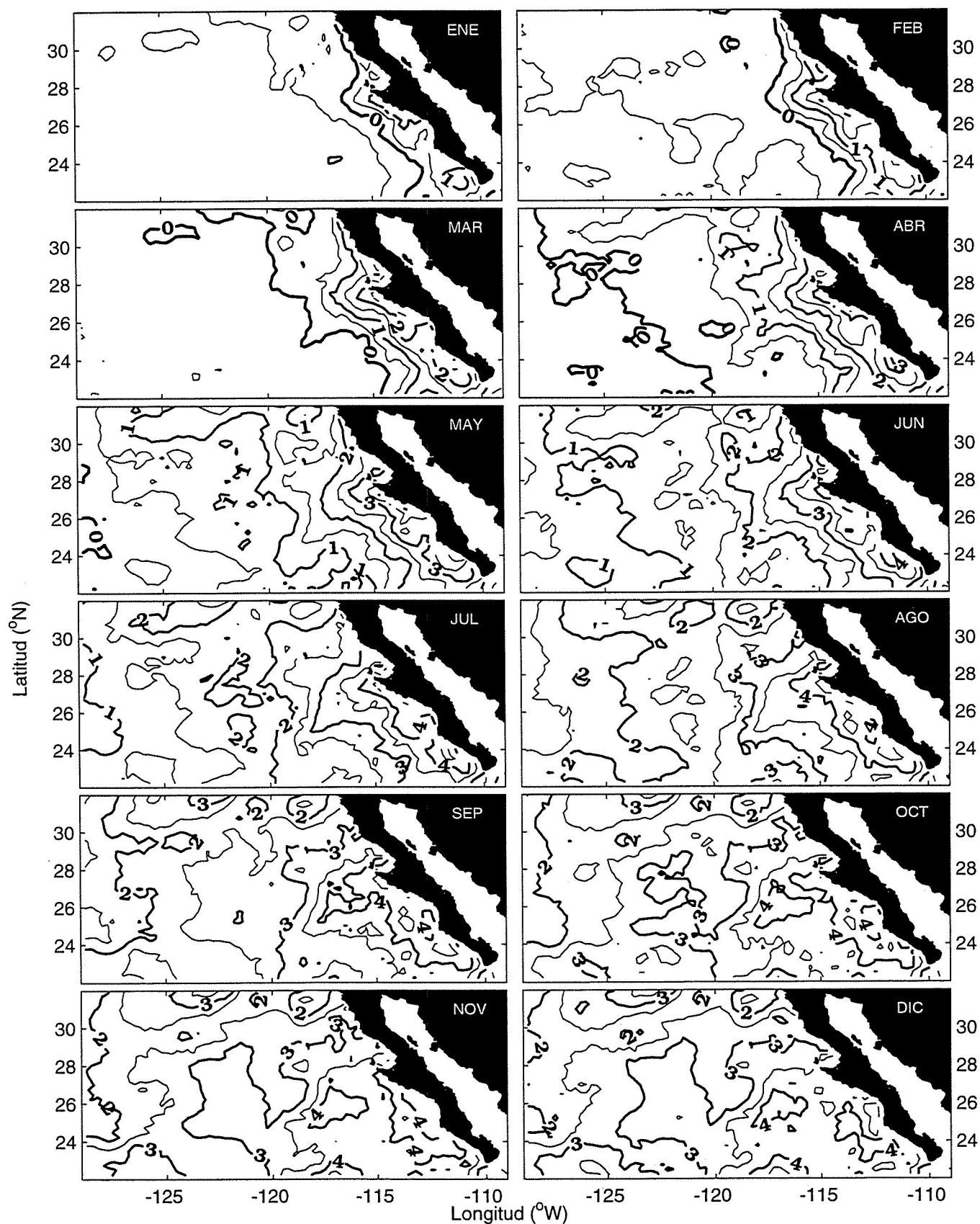
Figura 14.7- Anomalías termales interanuales para 1992
