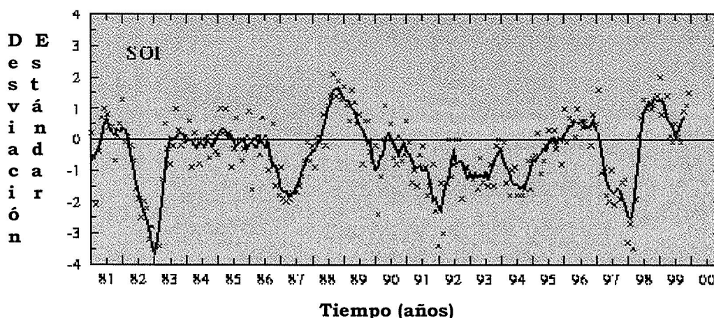
Figura 1. Índice de Oscilación del Sur (SOI, por sus siglas en inglés) para el área geográfica comprendida entre 5°N y 5°S, 160°E y -160°W.
