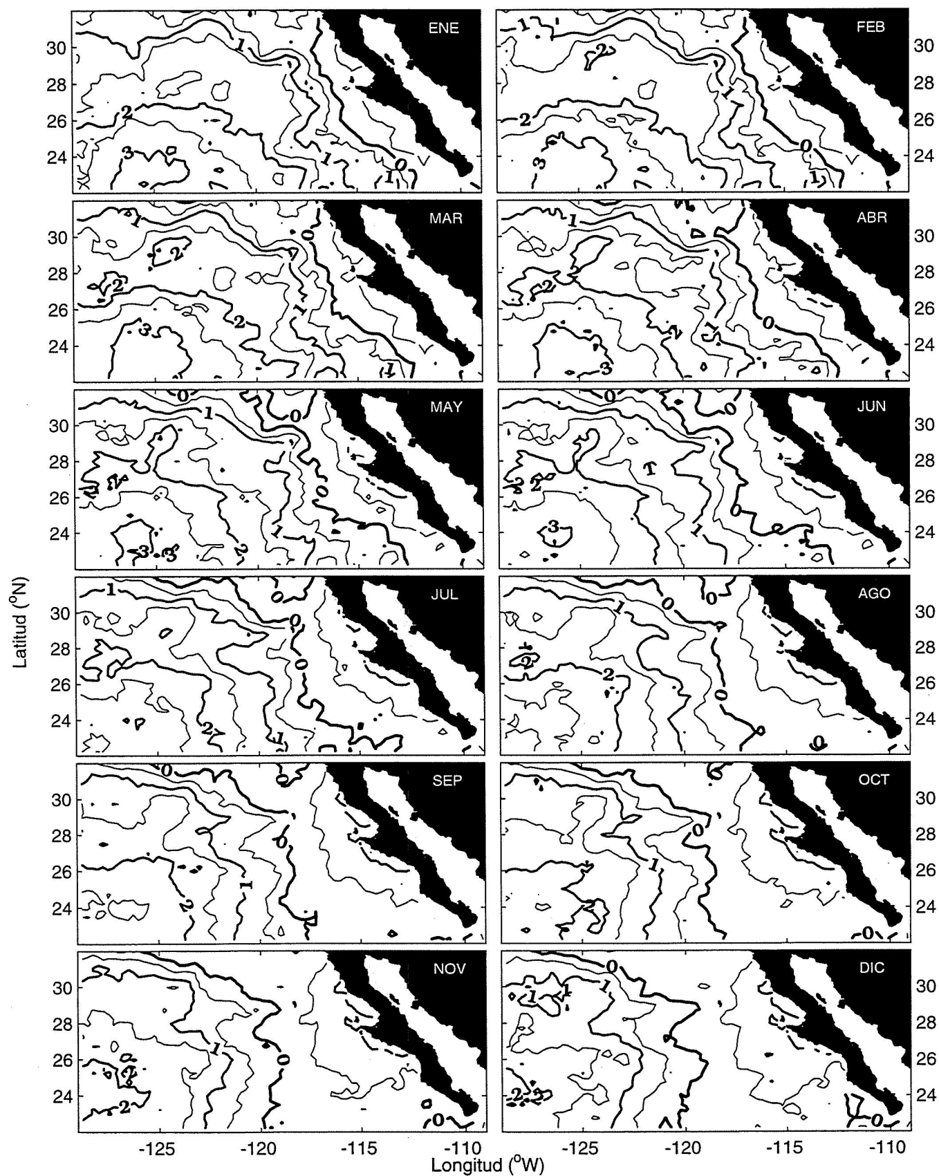
Figura 14.3- Anomalías termales interanuales para 1986
