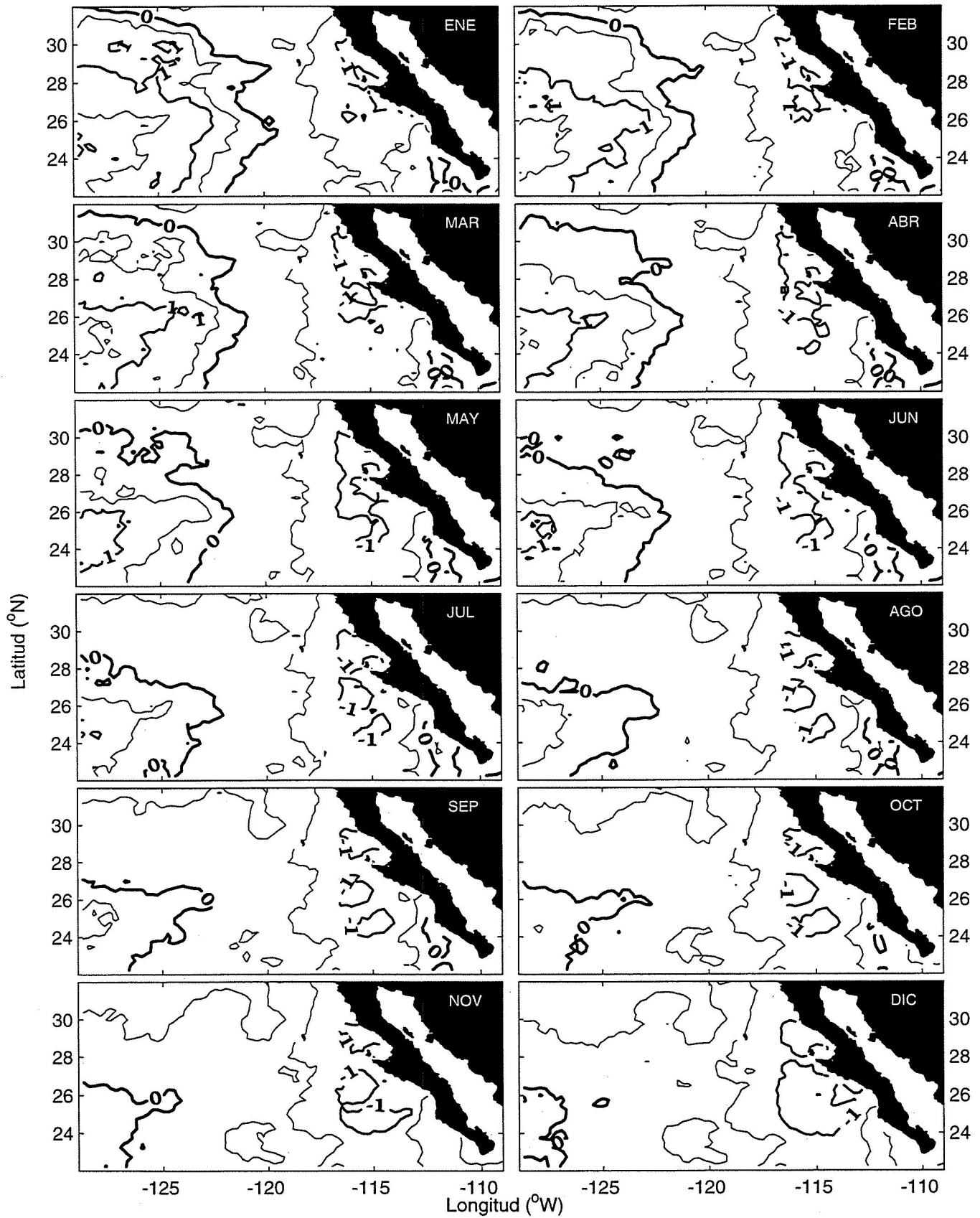
Figura 14.4- Anomalías térmicas interanuales para 1987
