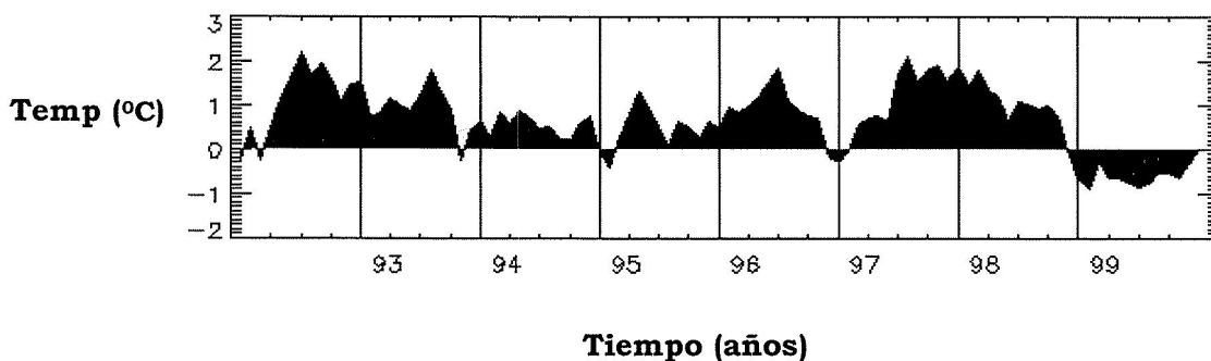
Figura 2. Anomalías de temperatura superficial para la región sur de California (30 a 35°N, 125 a 115°W).
