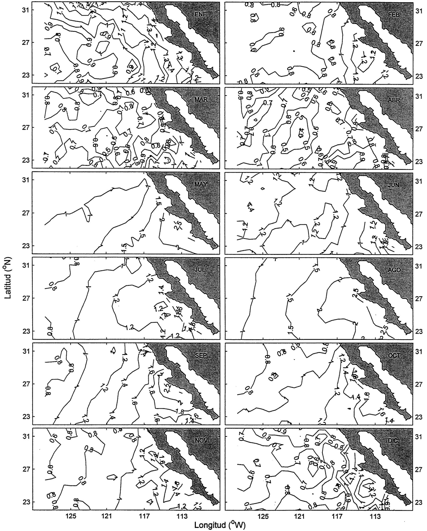
Figura 7. Desviación estándar del promedio climatológico mensual.
