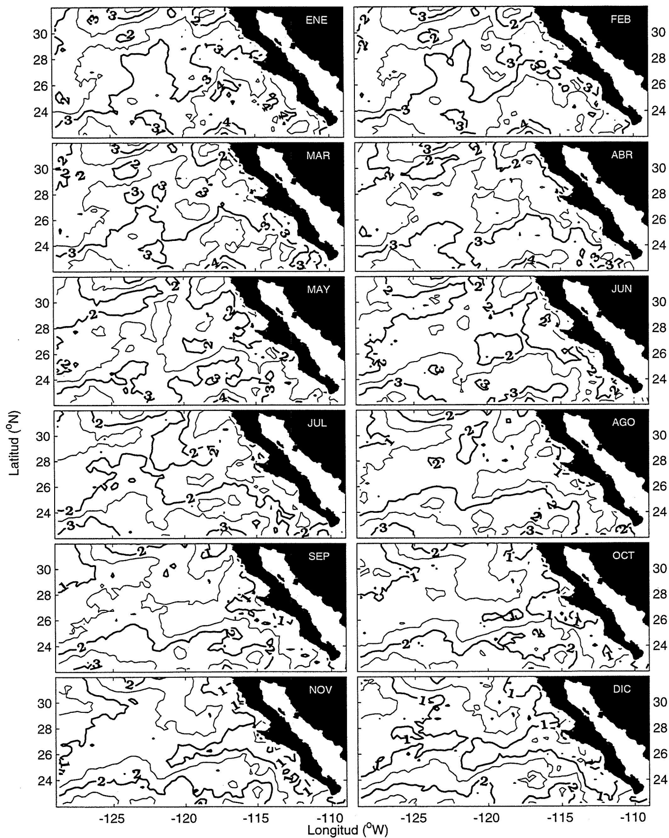
Figura 14.8- Anomalías térmicas interanuales para 1993
