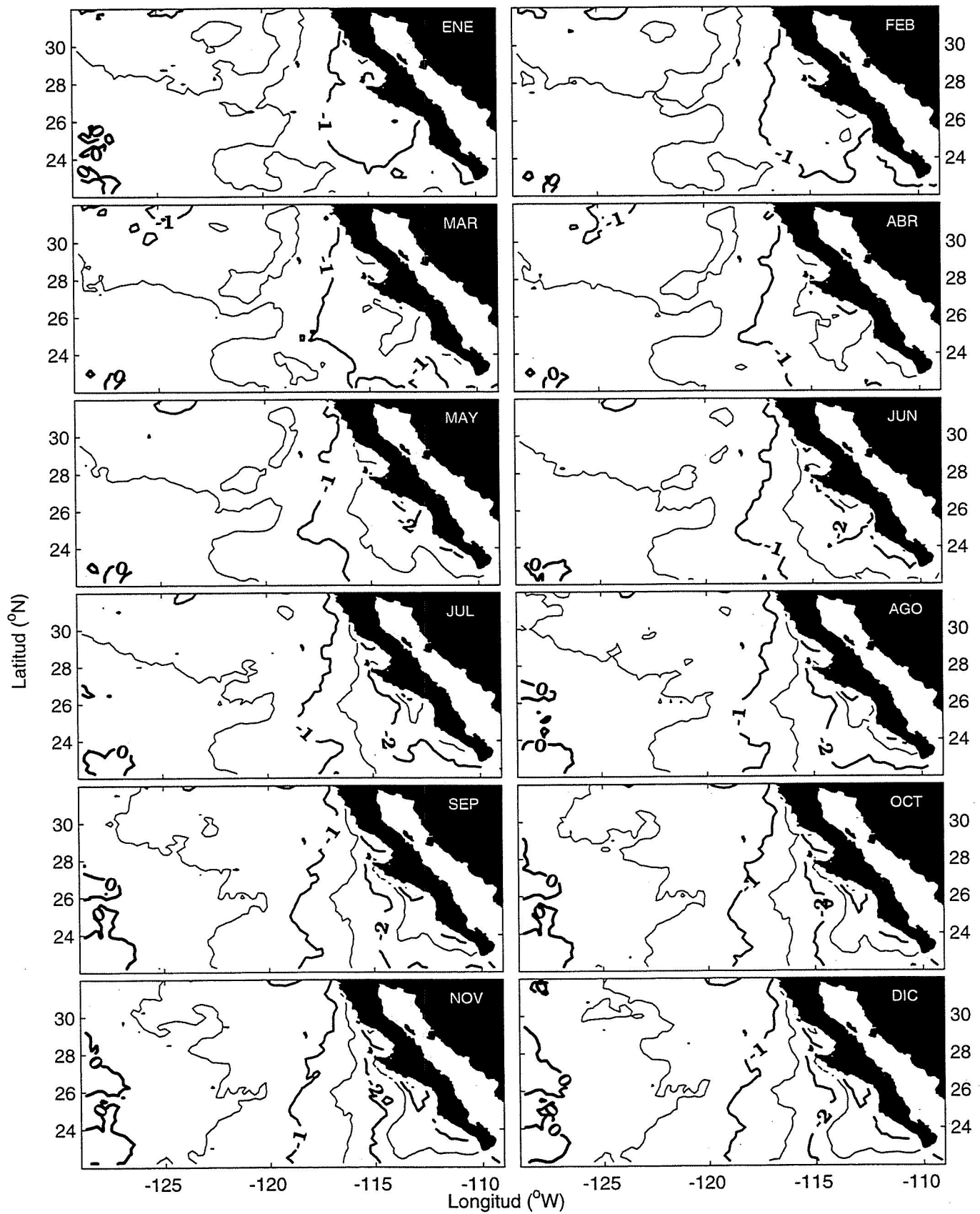
Figura 14.5- Anomalías térmicas interanuales para 1988
