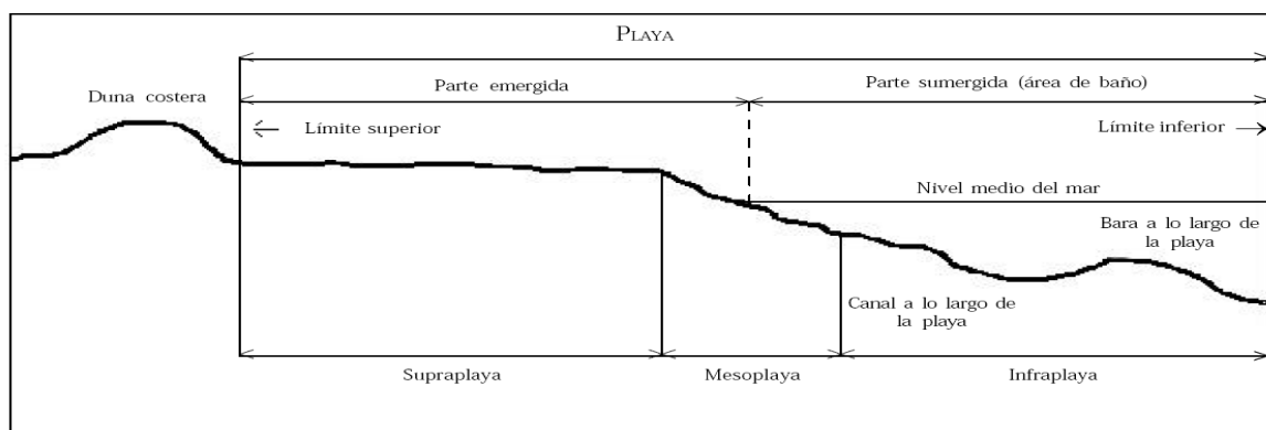
Figura 3. Descripción generalizada de un perfil de playa.
