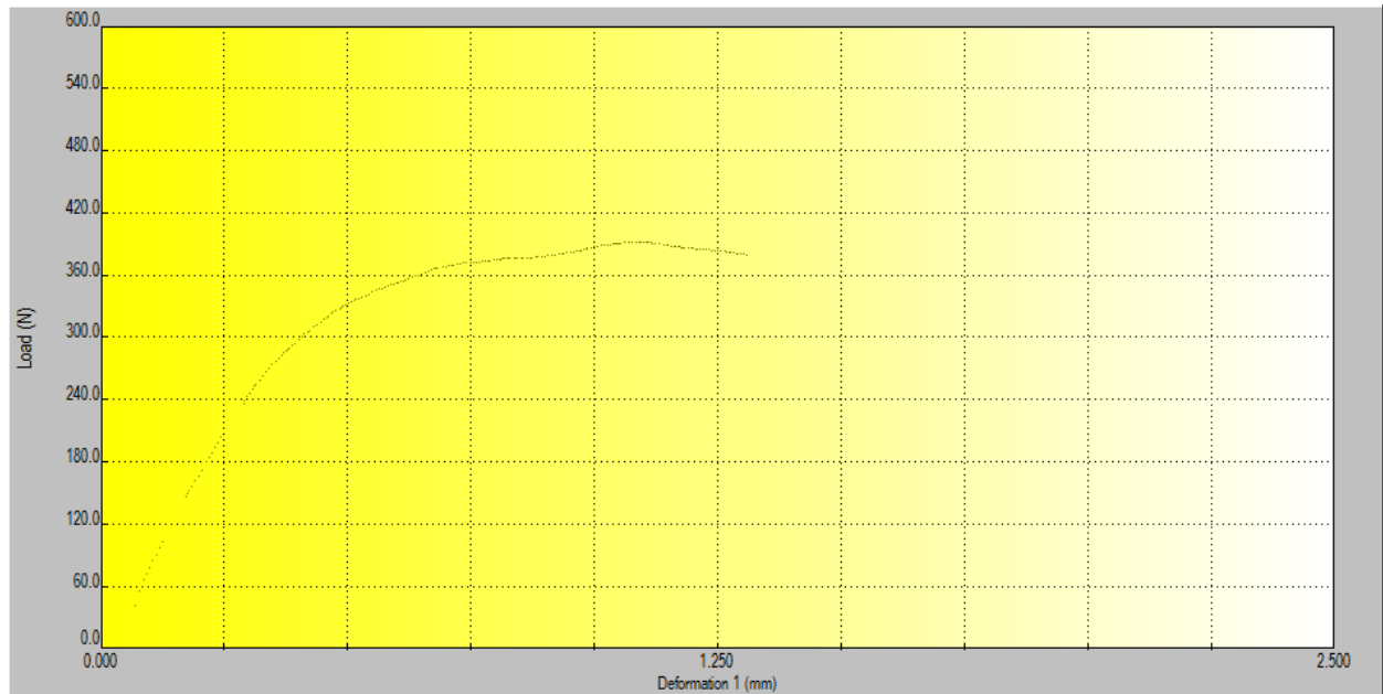
Gráfica 11. Fibras al 70% agua/ 30% solución (exposición al tratamiento de 5 minutos) Prueba 2.
