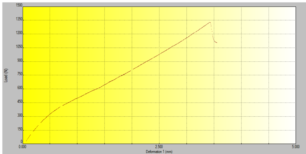
Gráfica 6. Fibras al 70% agua/ 30% solución (exposición al tratamiento de 30 minutos)- Prueba 1.
