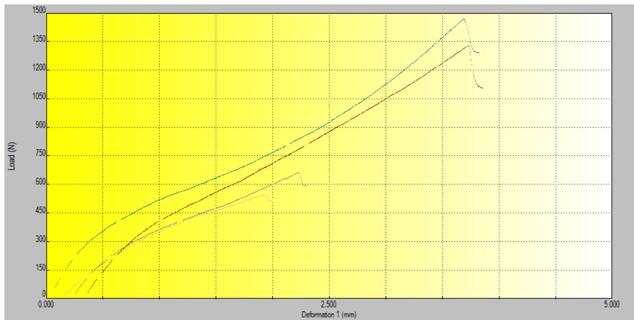
Gráfica 14. Imagen comparativa del tratamiento alcalino con 30 minutos de exposición.
