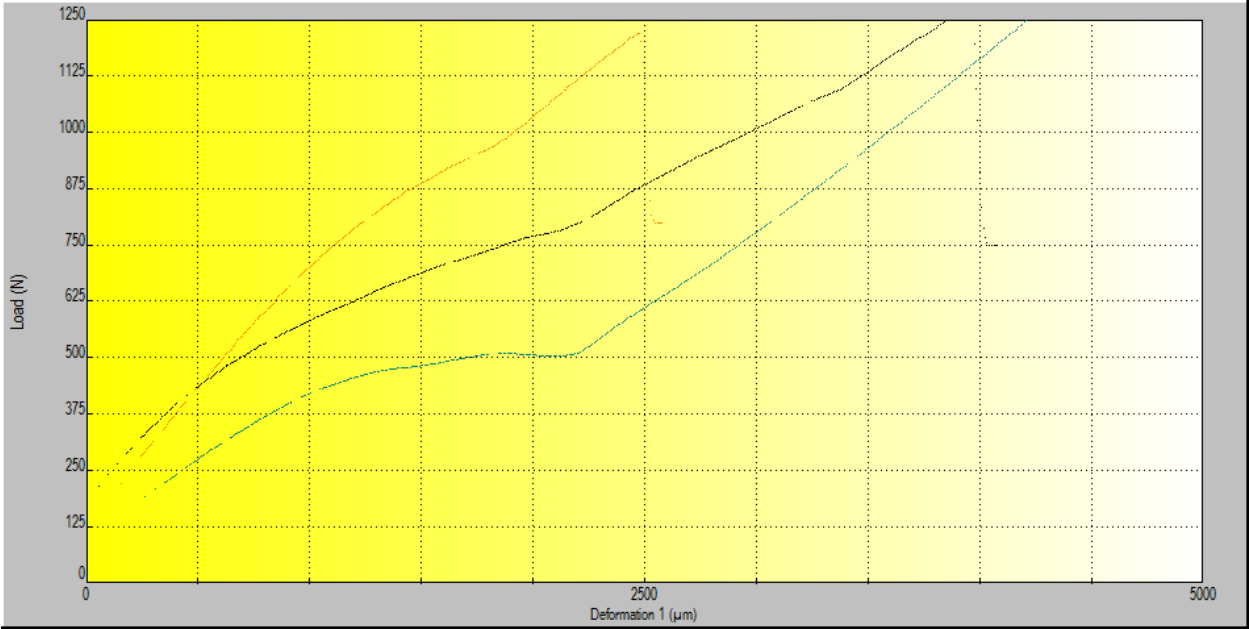
Gráfica 4. Comparativa de Fibras al 70% agua/ 30% solución.
