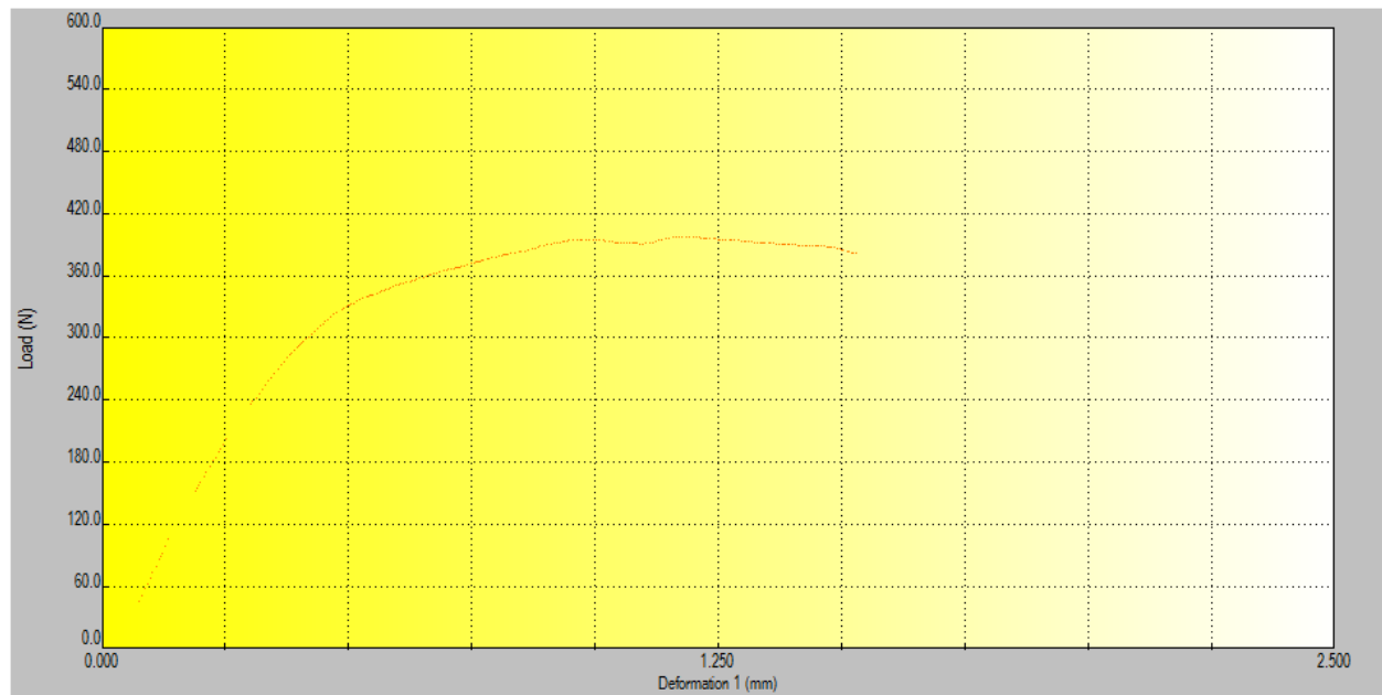
Grafica 12. Fibras al 70% agua/ 30% solución (exposición al tratamiento de 5 minutos) Prueba 3.
