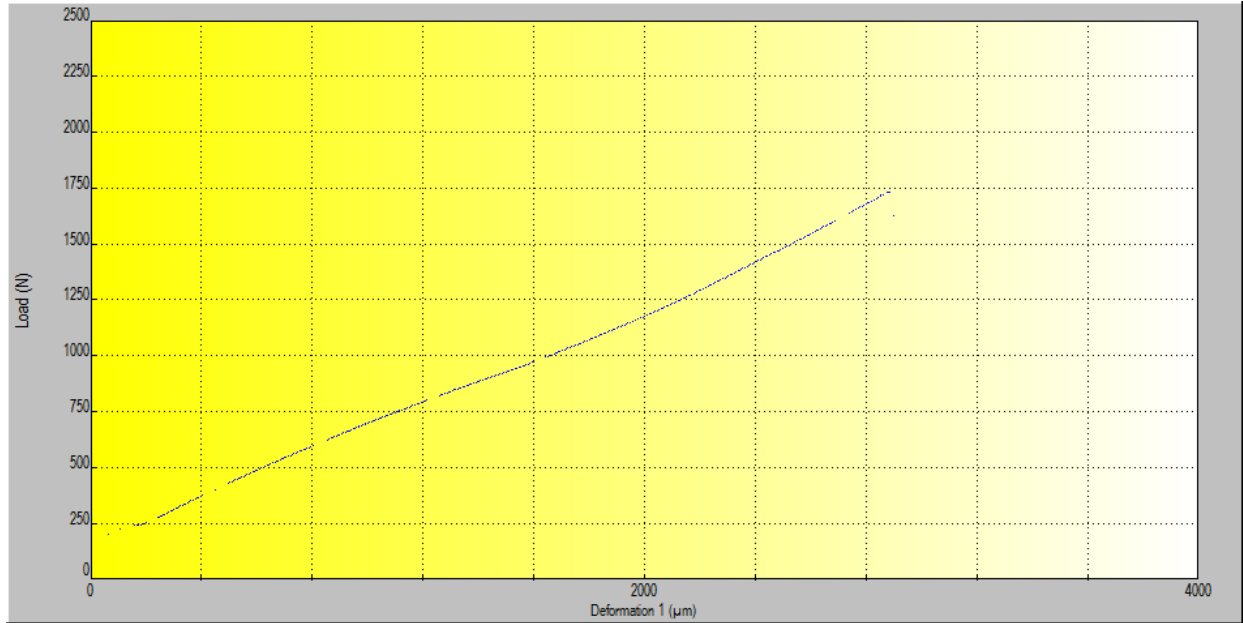
Gráfica2. Ejemplo de prueba de fibra sin tratamiento- resina epoxi.
