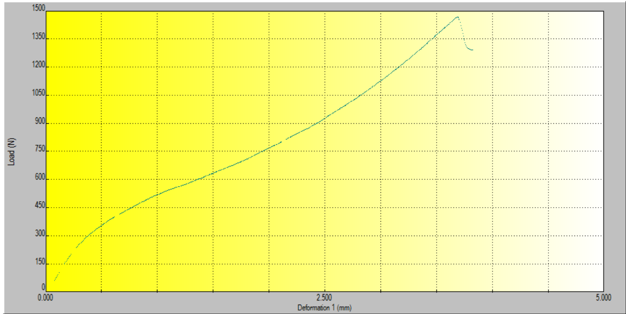
Grafica 9. Fibras al 70% agua/ 30% solución (exposición al tratamiento de 30 minutos) Prueba 4.
