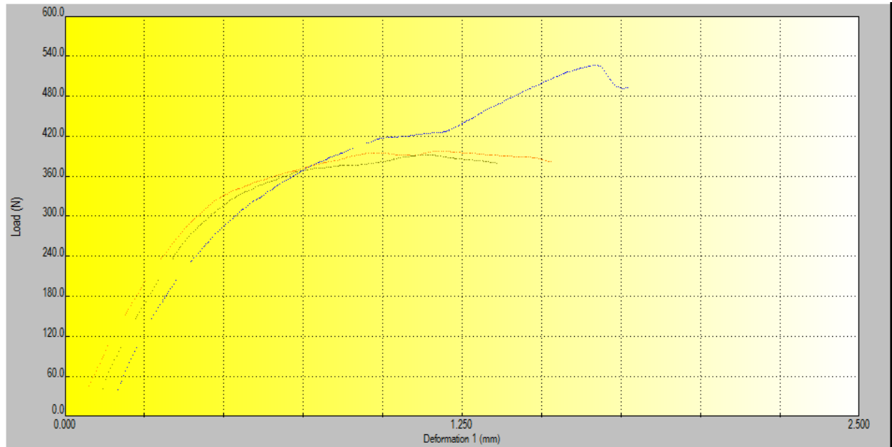
Gráfica 13. Imagen comparativa del tratamiento alcalino con 5 minutos de exposición.
