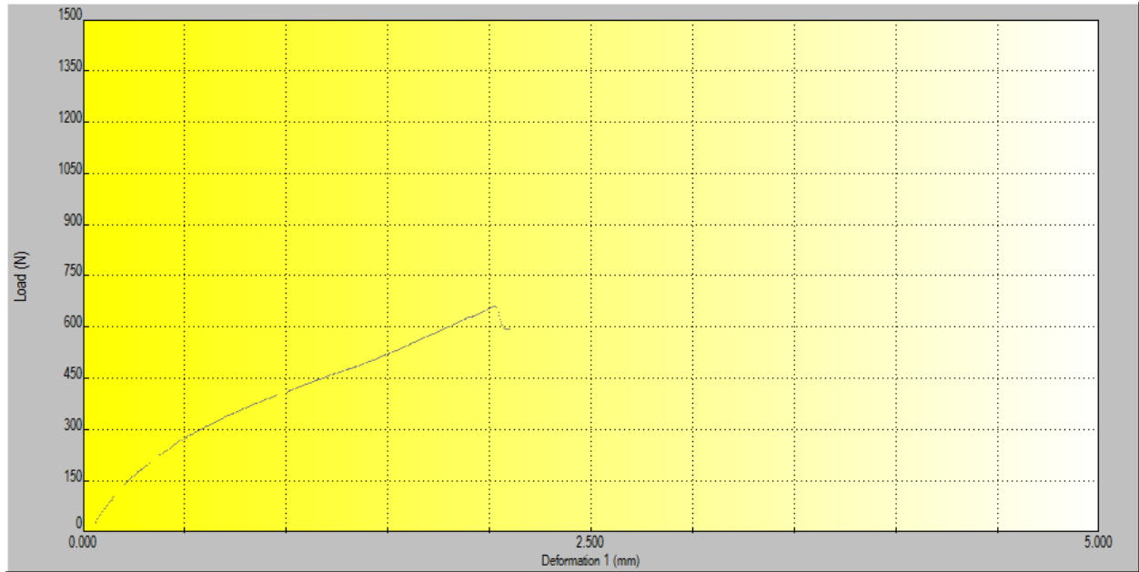
Gráfica 7. Fibras al 70% agua/ 30% solución (exposición al tratamiento de 30 minutos) Prueba 2.
