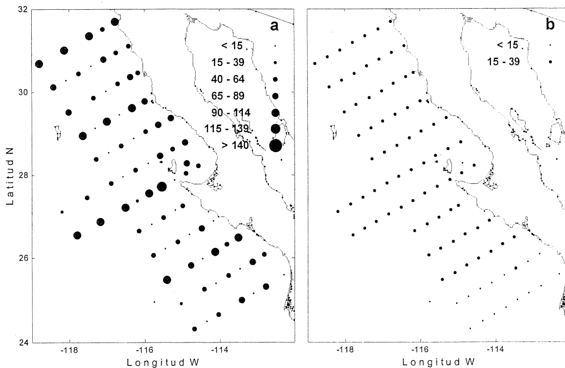
Figura 2.1 Número de ocupaciones de las estaciones oceanográficas de la región IMECOCAL para los períodos que comprenden: a) 1950-1978 (CalCOFI) y b) 1997-2004 (IMECOCAL).
