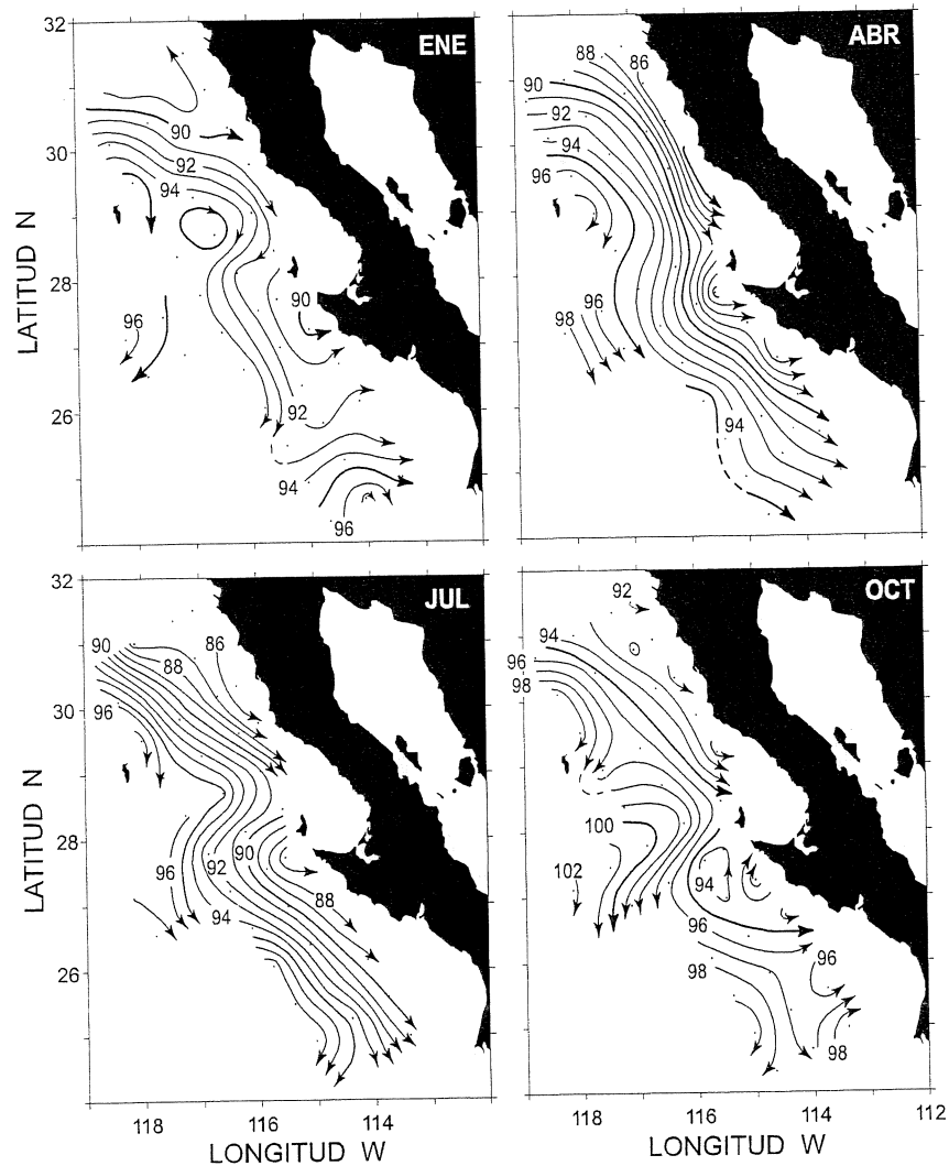
Figura 4.2. Altura dinámica en la superficie del mar relativo a 500 dbar. Intervalo de contornos de 1 cm din ( 1 \text{ cm din} = 0.01 \text{ J kg}^{-1} ). La dirección de la corriente esta indicada por las flechas.
