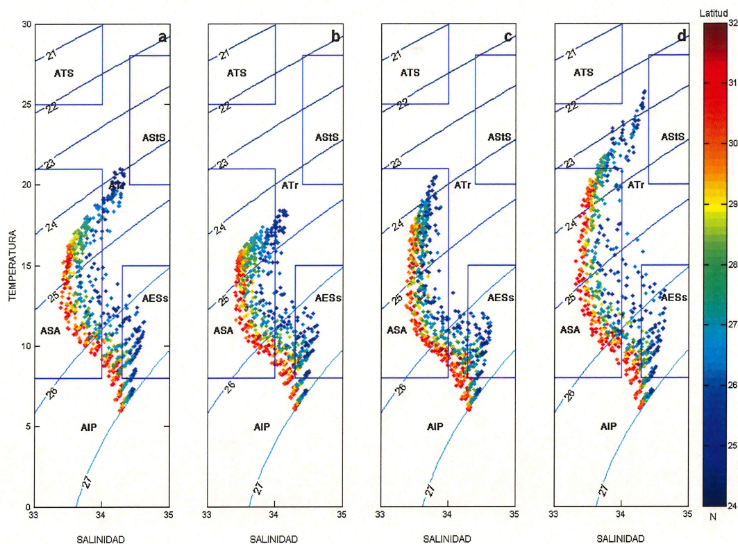
Figura 4.4 Diagramas T-S climatológicos del mes de a) enero, b) abril, c) julio y d) octubre. Agua Tropical Superficial (ATS), Agua Subtropical Superficial (AStS), Agua Transicional (ATr), Agua Subártica (ASA), Agua Ecuatorial Subsuperficial (AESs) y Agua Intermedia del Pacífico (AIP). La barra de colores indica la latitud de los datos. Rangos tomados de Durazo y Baumgartner (2002).
