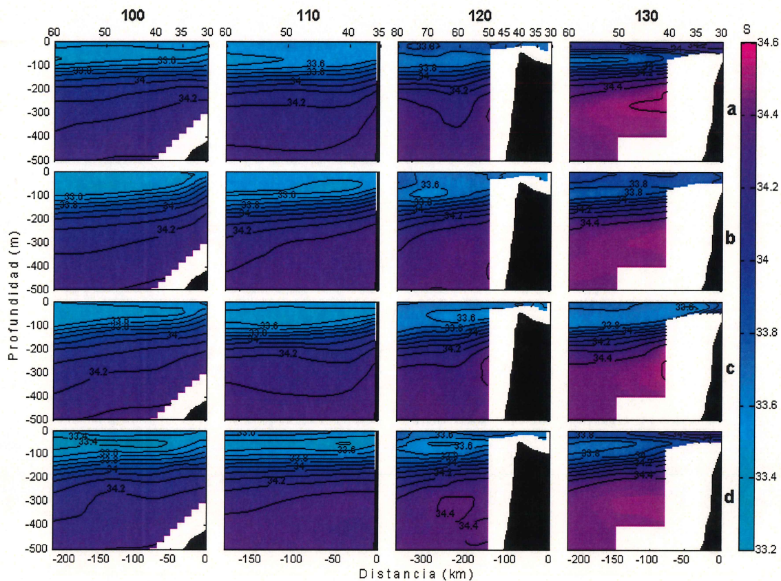
Figura 4.6. idem figura 4.5 para salinidad.
