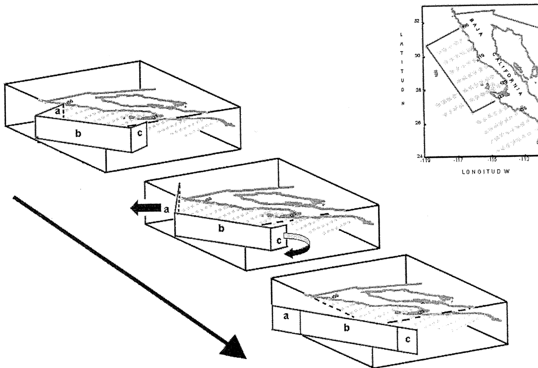
Figura 3.1 Caja control vista superficial. a) Cara norte formada por la línea 100, b) Cara oeste formada por las estaciones 60 y c) Cara sur formada por la línea 123.
