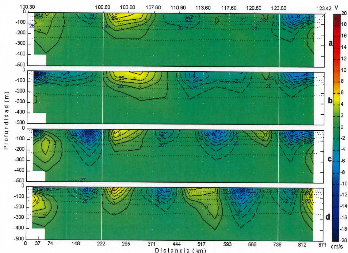
Figura 4.11 Velocidad geostrófica a través de la caja control calculada a partir de la climatología CalCOFI-IMECOCAL de temperatura y salinidad, a) enero, b) abril, c) julio y d) octubre. La convención de signos es: sobre la línea 100 y 123 una velocidad positiva (negativa) indica un flujo hacia el norte (sur) y sobre la línea paralela (estaciones 60) a la costa un valor positivo (negativo) indica un flujo hacia el este (oeste). La línea segmentada representa velocidad geostrófica negativa, línea continua velocidad geostrófica positiva y línea punteada indica contornos de \sigma_t .
