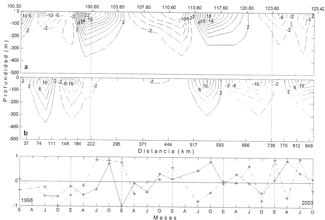
Figura 4.14 idem figura 4.12 para velocidad geostrofica.
