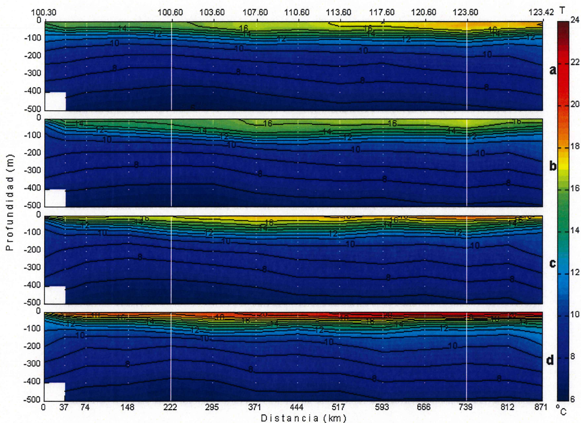
Figura 4.9 Climatología de temperatura de caja control a) enero, b) abril, c) julio y d) octubre. Los números en la parte superior representan la línea-estación. Las líneas verticales indican las esquinas de la caja. El intervalo de contornos es de 1^{\circ}\text{C} .
