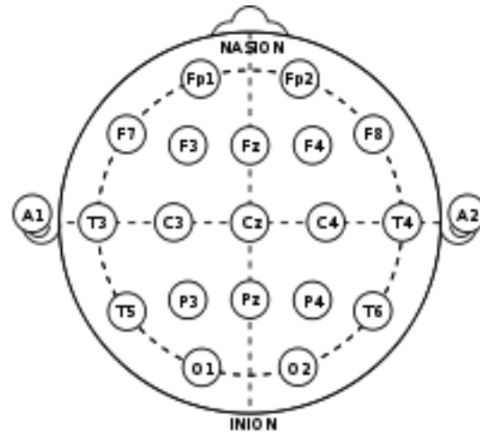
Figura 2.4: Sistema Internacional 10-20.
