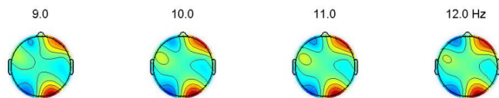
Figura 3.12: Espectro de la onda cerebral Alfa.
